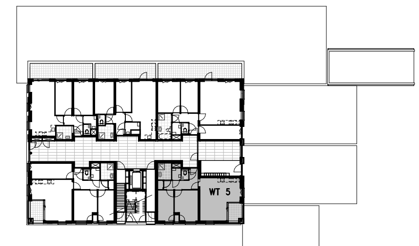
Begane grond
